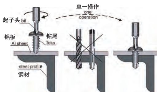
Fig.5 An Example of Using Tek Screws 图五 Tek 钻尾螺丝应用实例之一
